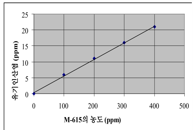
이론적인 교정 차트 M-615 vs 유기인산염 농도:
